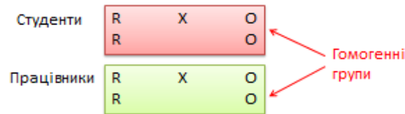
Рис. 10.5. Дизайн випадкових блоків
